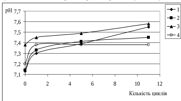
Рис. 1. Залежність значень рН водопровідної води від кількості циклів кавітаційної обробки при діаметрі горловини змінного кавітаційного реактора.
