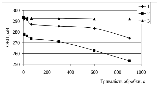
Рис. 4. Залежність ОВП водопровідної води від тривалості кавітаційної обробки в кавітаційному змішувачі при діаметрі горловини сопла змінного кавітаційного реактора 0,012 м.
