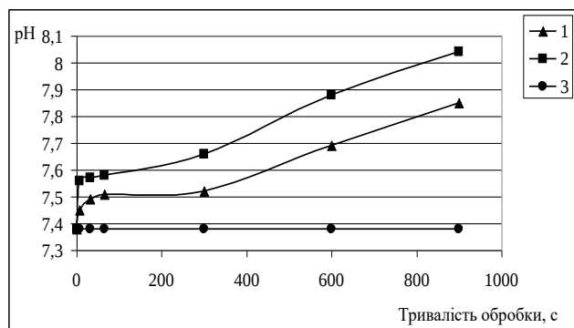
Рис. 2. Залежність значень рН водопровідної води від тривалості кавітаційної обробки в кавітаційному змішувачі при діаметрі горловини змінного кавітаційного реактора 0,012 м.
