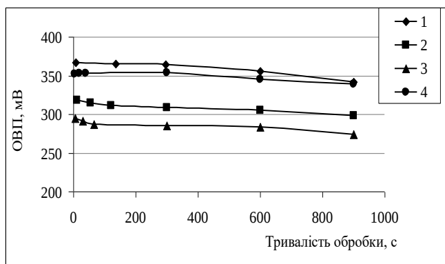
Рис. 3. Залежність значень ОВП водопровідної води від тривалості кавітаційної обробки при діаметрі горловини змінного кавітаційного реактора.
