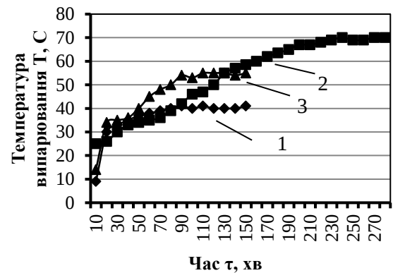
Рис. 5 Термограми процесів випарювання.
