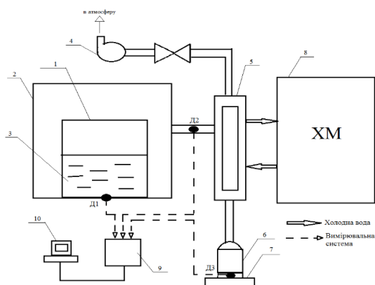
Рис. 1. Експериментальний стенд мікрохвильової випарної установки.
