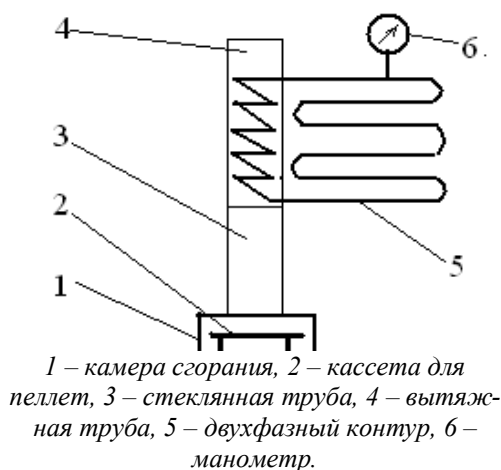
Рис. 1 – Экспериментальный стенд
