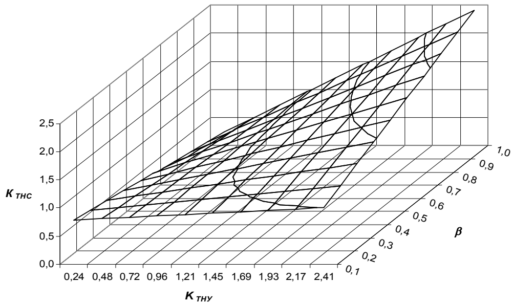
Рис. 1 – Значення безрозмірного критерію енергетичної ефективності ТНС з електричним приводом для випадків змінного навантаження ТНУ, за умови споживання електроенергії з енергосистеми України
