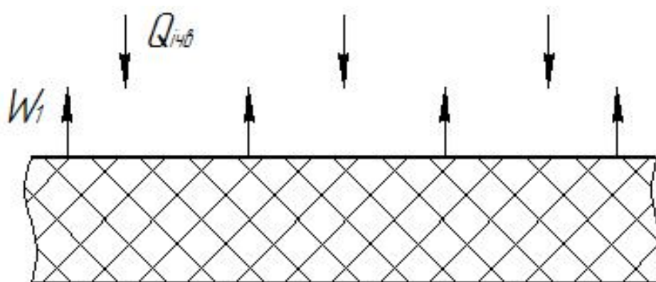
Рис. 2 – Схема випаровування води з вільної поверхні матеріалу
