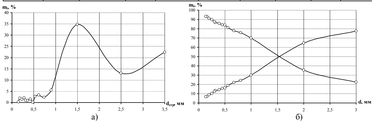
Рис. 2 – Диференціальна (а) та інтегральна (б) крива розподілу подрібненої рослинної зернової сировини (кукурудза, крупний помол)
