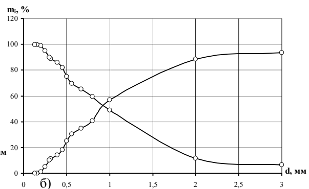
Рис. 5 – Диференціальна (а) та інтегральна (б) крива розподілу подрібненої рослинної зернової сировини (пшениця, дрібний помол)
