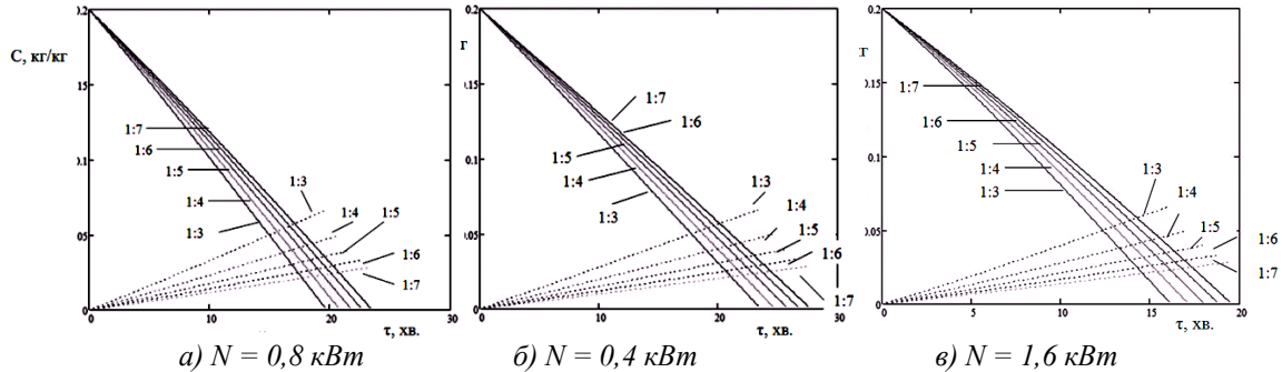
Рис. 5 – Зміна концентрації (%) цільового компонента в рідкій (пунктирні лінії) і твердій (суцільні лінії) фазі з плином часу (хв.).
