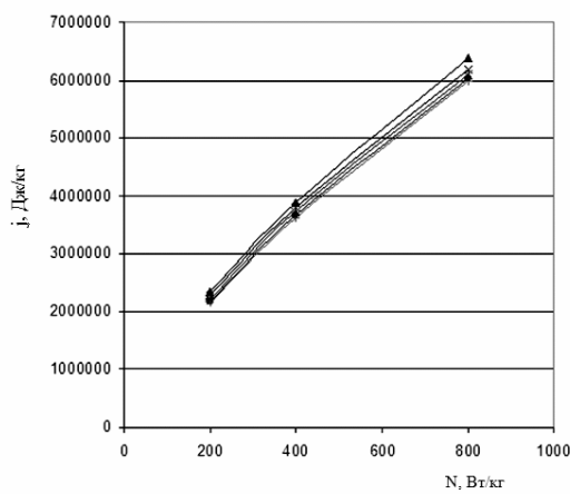
Рис. 7 – Залежність питомого енергоспоживання (Дж/кг перенесеної речовини) від питомої потужності НВЧ випромінювача (Вт/кг сировини) при різних значеннях гідромодуля
