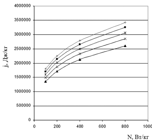
Рис. 4 – Залежність питомого енергоспоживання (Дж/кг перенесеної речовини) від питомої потужності НВЧ випромінювача (Вт/кг сировини) при різних значеннях гідромодуля.
