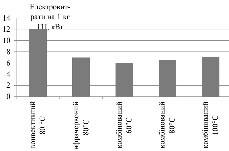
Рис. 5 – Залежність витрат енергії на сушіння глоду від температури теплоносія при різних методах
