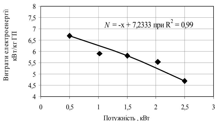
Рис. 6 – Залежність витрат енергії від потужності темних тенів при комбінованому методі енергопідведення, кВт/кг готового продукту
