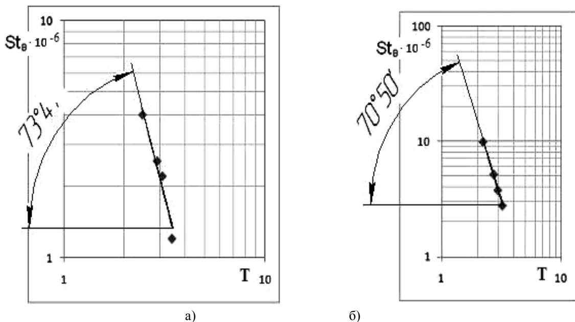
Рис. 3 – Графік залежності модифікованого вібраційного числа Стантона від безрозмірної температури ( T=T_n/T_o ); а) завантаження контейнера \Pi=0,67 ; б) завантаження контейнера \Pi=0,5
