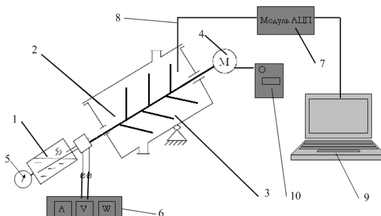
1 – парогенератор; 2 – конденсатор; 3 – корпус; 4 – привод; 5 – манометр; 6 – измерительный комплекс K-50; 7 – АЦП; 8 – термопары; 9 – компьютер; 10 – частотный преобразователь
