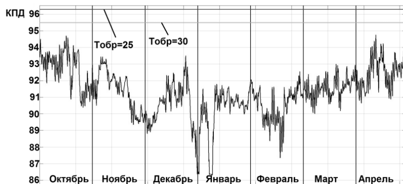
Рис. 4 — Изменение КПД КГВК в течение отопительного сезона
