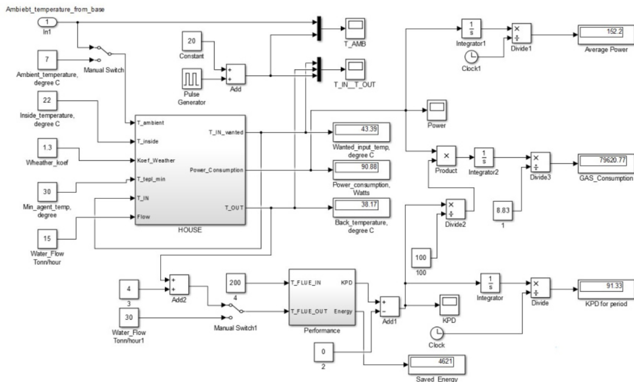
Рис. 1 — Блок—схема модели для оценки эффективности КГТА
