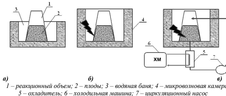
Рис. 1 – Экспериментальные стенды
