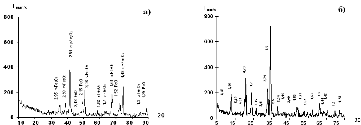
a – повітряна окалина; б – \text{Na}_2\text{H}_2\text{P}_2\text{O}_7 + 20% повітряної окалини
