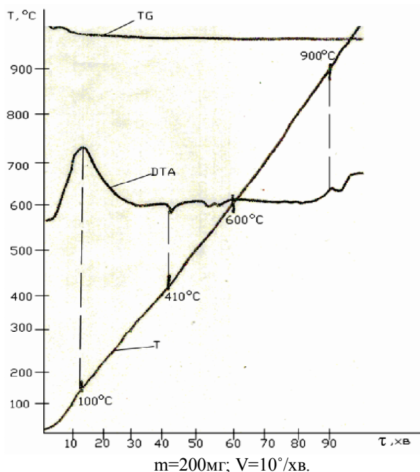
Рис. 2 – Термограма модельної системи «повітряна» окалина (20 % мас.) – натрій пірофосфат
