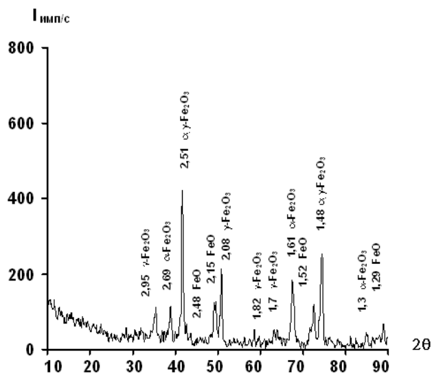
Рис. 1 – Рентгенівська дифрактограма повітряної окалини
