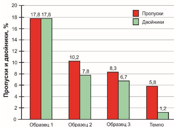
Рис. 1 – Средненные результаты исследований точности высева разными сеялками
