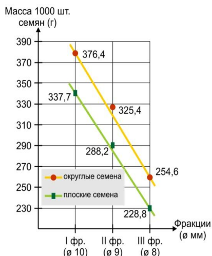
Рис. 7 - Зависимость массы 1000 шт. семян кукурузы (г) от формы семян кукурузы (округлые и плоские)
