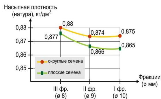
Рис. 9 - Насыпная плотность (натура) семян кукурузы разных размеров и формы (округлая и плоская)
