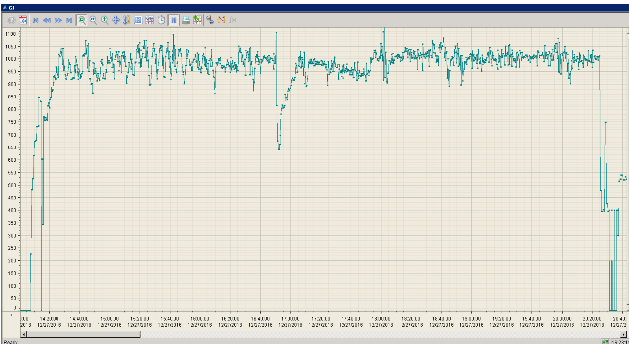
Рис. 6 – Фрагменты изменения производительности ПТЛ под управлением АСОЗ (Ca1.1), интервал времени 8 часов.
